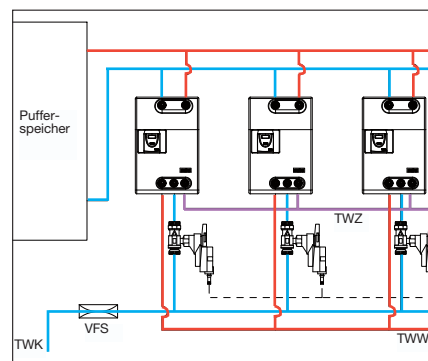
System-Darstellung
