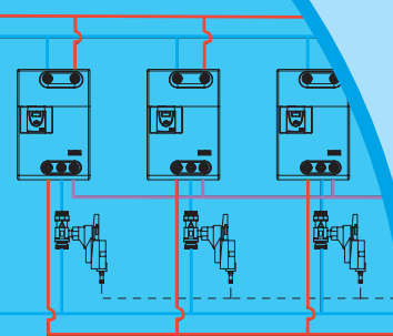
„Regumaq XK“ Kaskadierungs-Set
