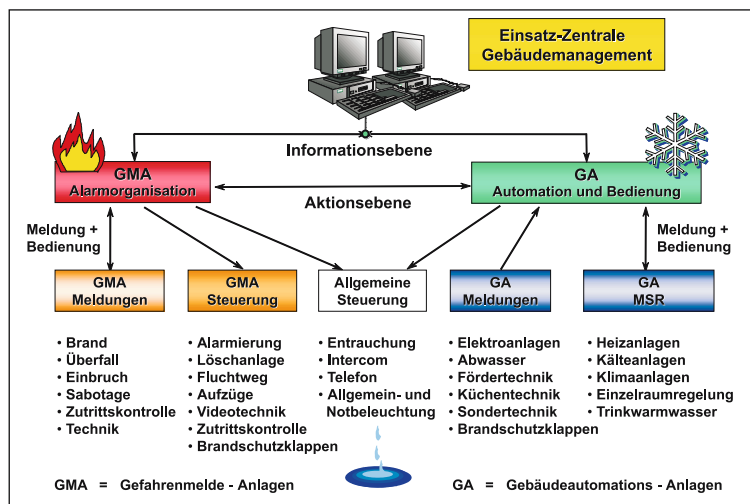
Bild 1 – Systemintegration (HAK).
