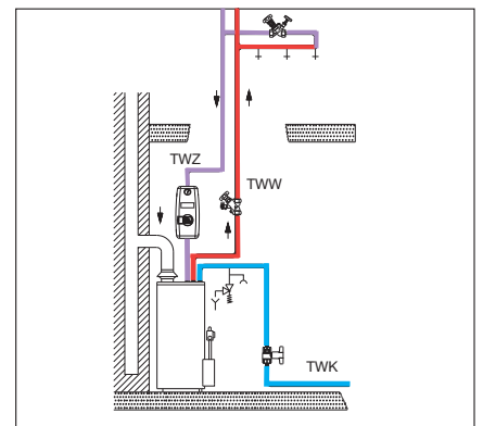
System-Darstellung
